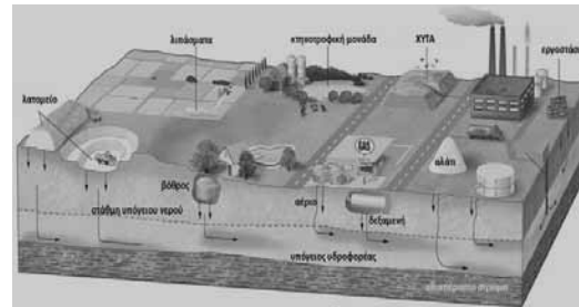
Εικ.3 Διάφορες πηγές ρύπανσης του υπόγειου νερού από ανθρώπινες δραστηριότητες (πάνω) και διαδικασίες αυτοκαθαρισμού σε υπό πίεση υδροφόρο ορίζοντα (κάτω).
