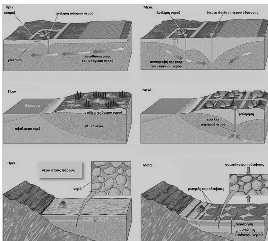
Εικ.2 Ρύπανση του υδροφορέα με αναστροφή της ροής(α,β), υφαλμύριση(σ,δ)και καταστροφή του πορώδους (ε,φ)
