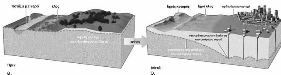
Εικ.1 Πριν(α) και μετά (β) την άντληση και την πώση της στάθμης του υδροφορέα
