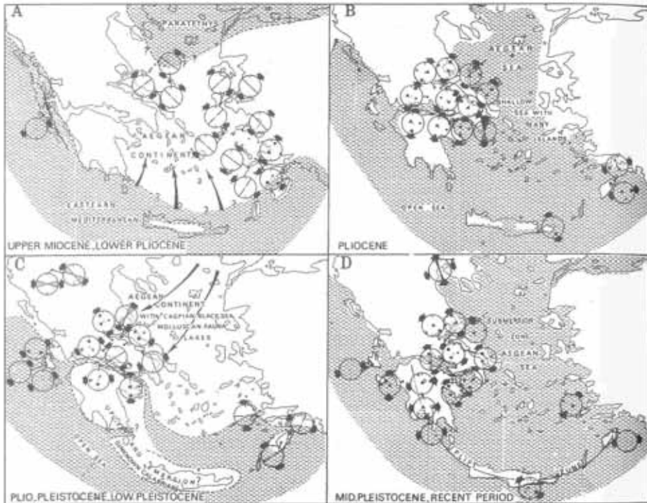
Σταδιακή αναπαράσταση της νεοτεκτονικής εξέλιξης και δημιουργίας του Ελλαδικού χώρου από το Ανώτερο Μειόκαινο μέχρι σήμερα (κατά Mercier 1977)
