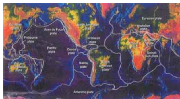
Το παγκόσμιο σύστημα των λιθοσφαιρικών πλακών με απεικόνιση του ωκεάνιου και ηπειρωτικού τμήματος της κάθε πλάκας
