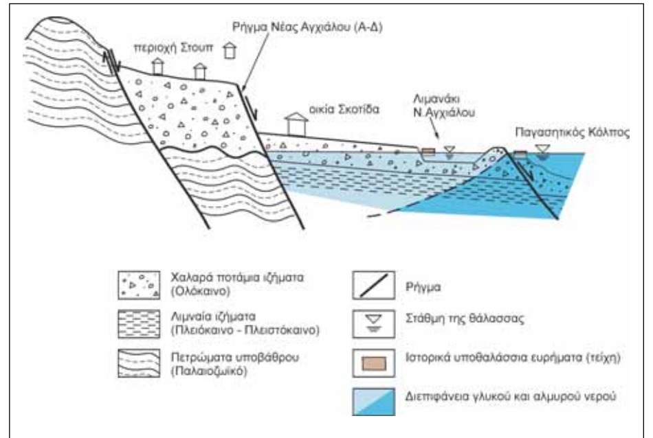
Γεωλογικό σκαρίφημα του νεοτεκτονικού σχηματισμού της περιοχής της Νέας Αγχιάλου
